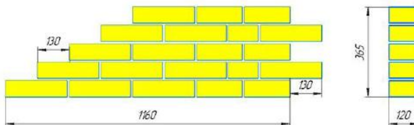
Общий вид модулей 1,2, вариант 1.
